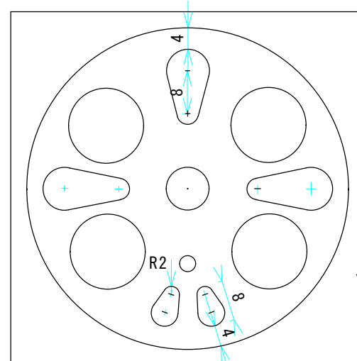
C バルサ材シート (厚さ1mm) 穴あけポンチで穴を開ける 4個
