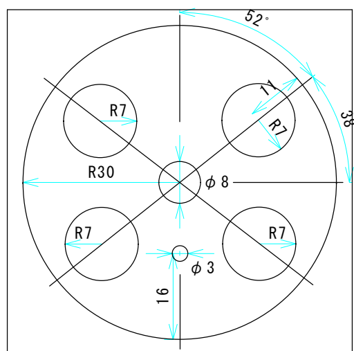
A バルサ材シート (厚さ3mm) 穴あけポンチで穴を開ける 6個
