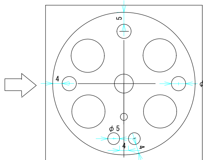
B バルサ材シート (厚さ1mm) 穴あけポンチで穴を開ける 4個
