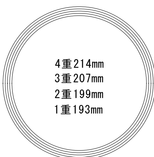
5本幅で4重に巻く シルバー
