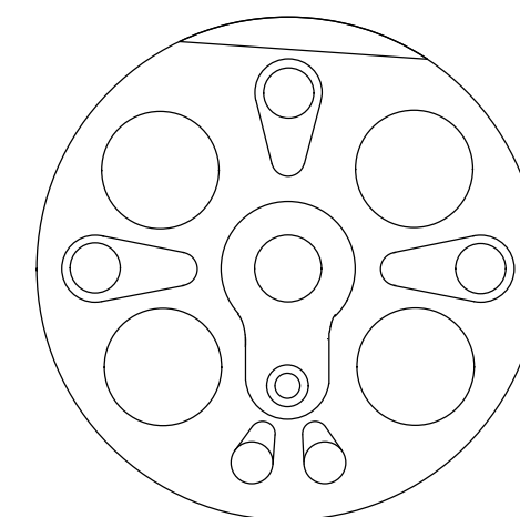
下からABCの順に貼り合わせる 電動丸ノコ盤で円形に切る 第一・三動輪 4個
