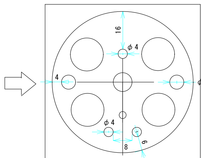
B バルサ材シート (厚さ1mm) 穴あけポンチで穴を開ける 2個
