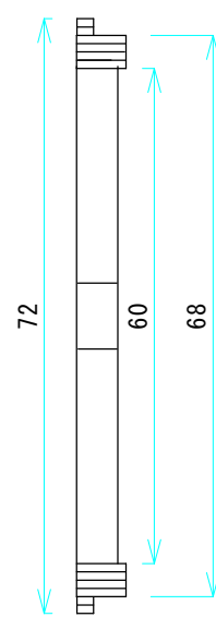
側面図
