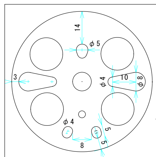
C バルサ材シート (厚さ1mm) 穴あけポンチで穴を開ける 2個
