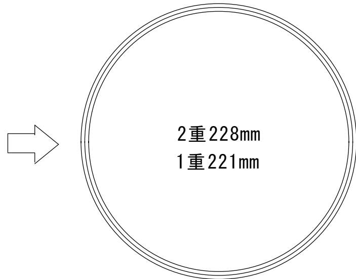
更に2本幅で2重に巻く シルバー
