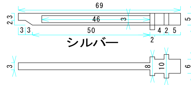
滑り棒
