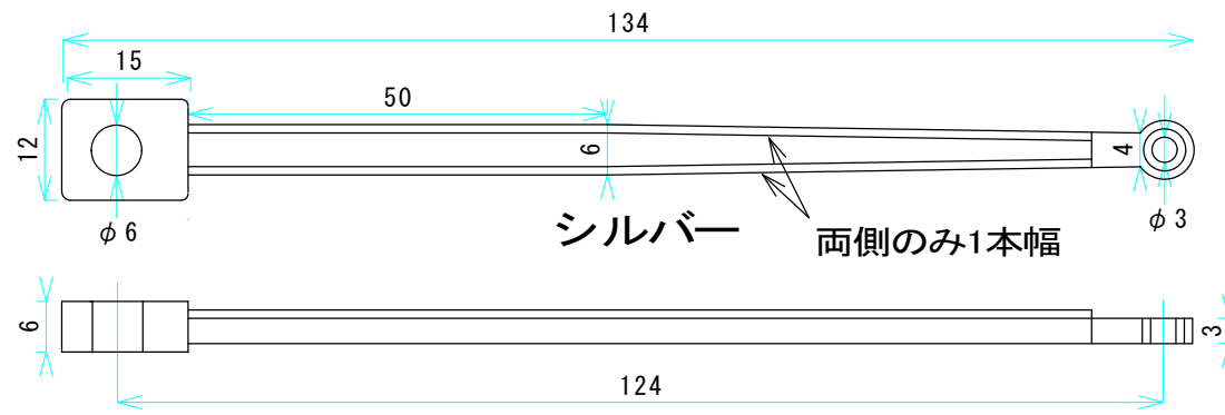
主連結棒
