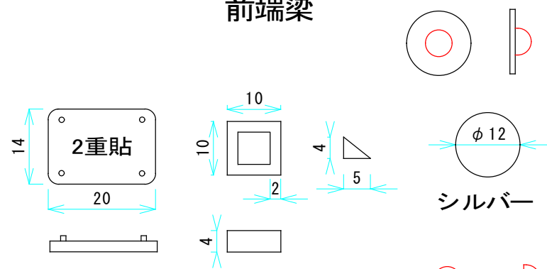
前端梁
